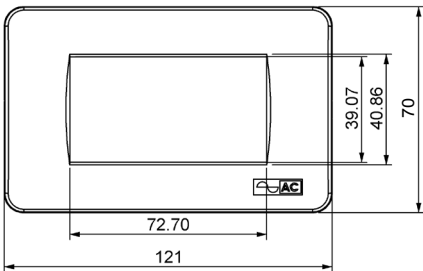
* Kích thước ngoài của các mặt AR1S, AR2S, AR3S
