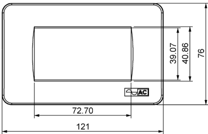
* Kích thước ngoài của các mặt AR1, AR2, AR3
