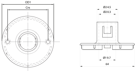
NẮP ĐẬY CÓ LỖ CHỈ DÀNH CHO ỐNG LUỒN ĐÀN HỒI Ø 20MM /PVC JUNCTION BOX COVER USED FOR CORRUGATED CONDUIT Ø 20MM
